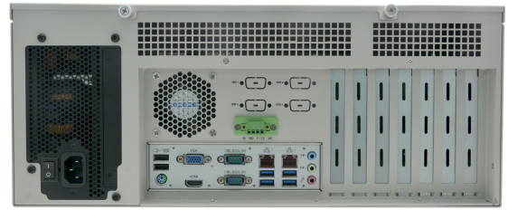
后置I/O视图
